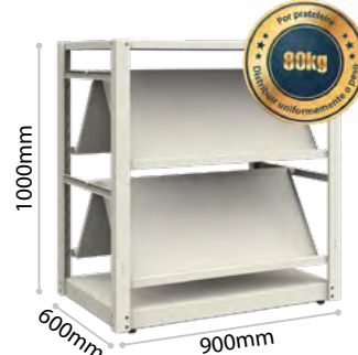
Estante Bibliotec Expositora Dupla - Mini Nk 2111
