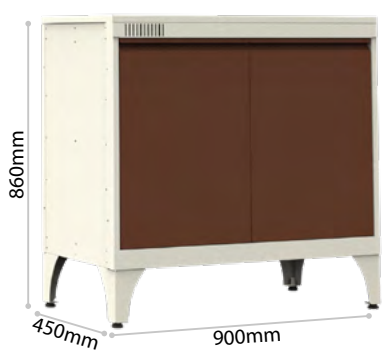
Armário Café Nk 1806 Tampo em Aço Galvanizado
