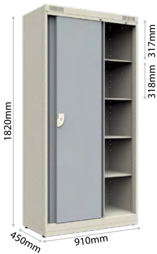
Armário Escritório Nk 1812 *Com porta de correr
