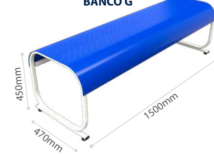
Nk 1906 BANCO G
