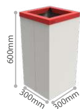
Nk 2003 SIMPLES - 50 LITROS
