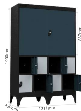
Nk 184491 ARMÁRIO CARREGADOR PARA FERRAMENTAS ELÉTRICAS
