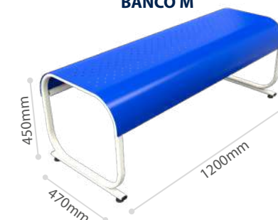
Nk 1907 BANCO M
