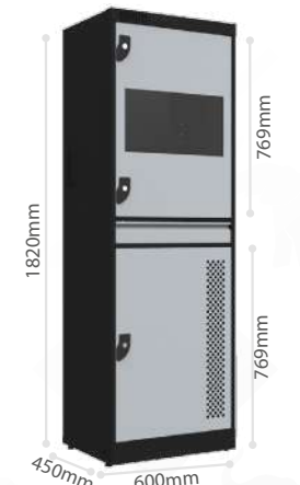
Nk 1713 RACK DE COMPUTADOR INDUSTRIAL
